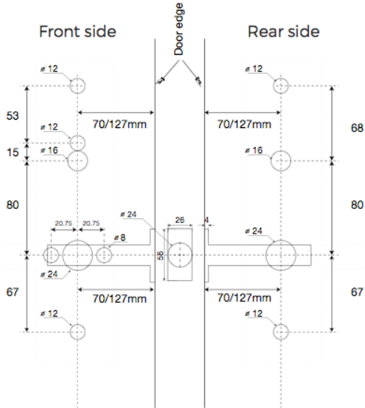
TL-Tubular Latch
